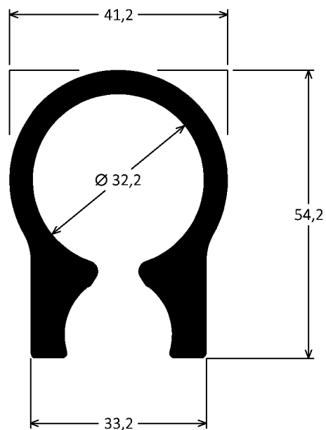
AP-026 2,040kg/m
