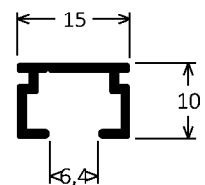
BK-299 0,144kg/m
