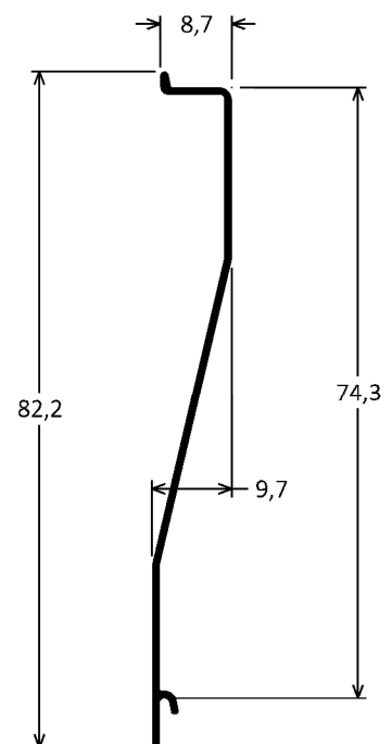
CX-078 0,230kg/m
