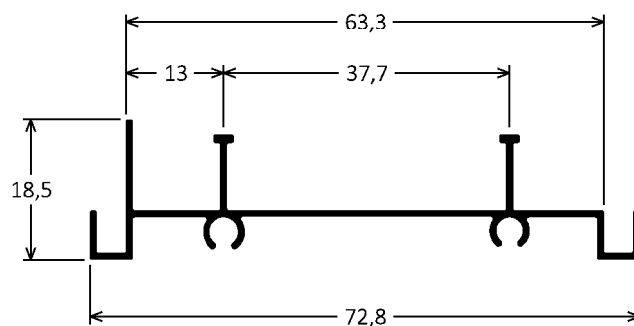
CX-484 0,357kg/m
