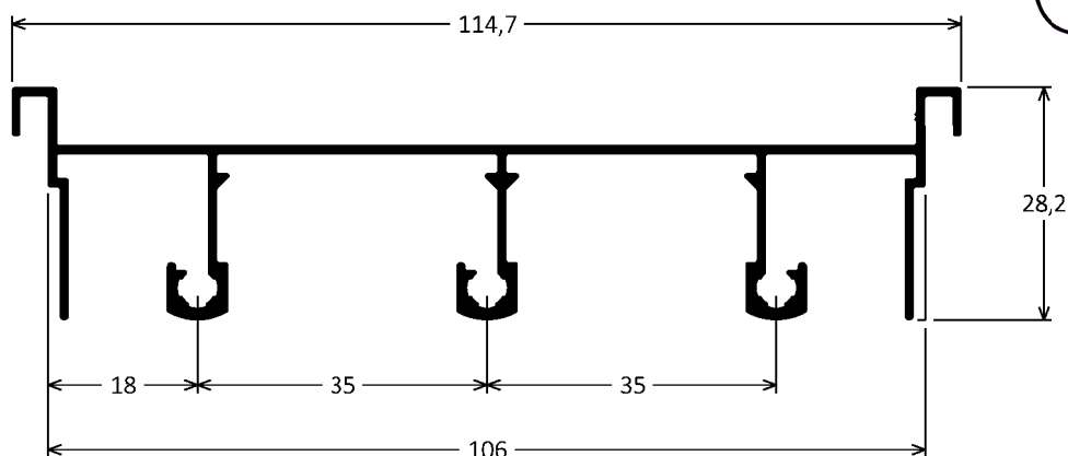
ISA-013 0,913kg/m
