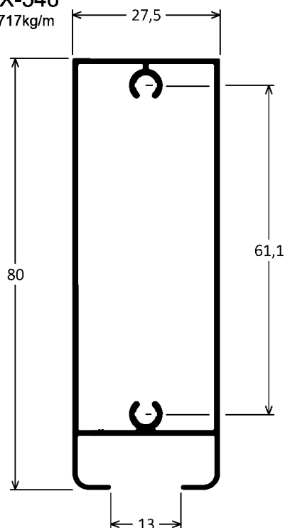
CX-545 0,661kg/m
