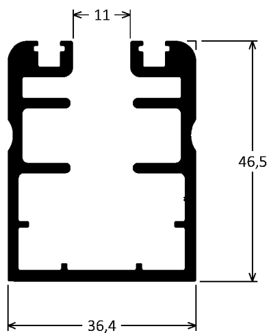
SKD-021 1,271kg/m
