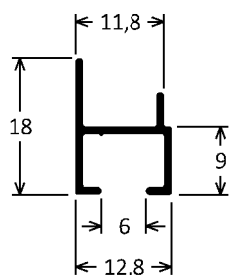
CX-084 0,126kg/m
