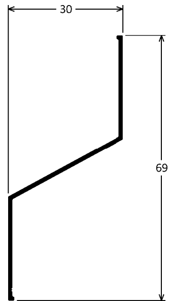
VZ-160 0,259kg/m
