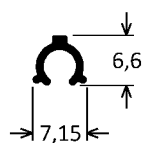
BK-665 0,047kg/m
