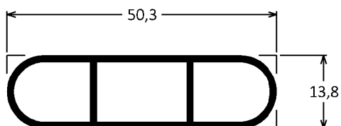
DV-058 0,474kg/m
