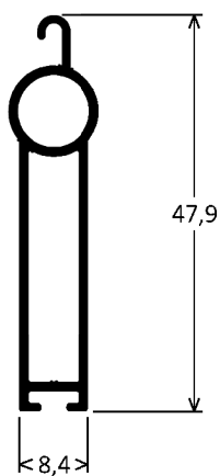
IMN-055 0,352kg/m
