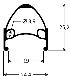
AP-085 0,266kg/m
