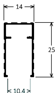
BX-012L 0,162kg/m
