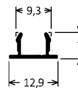
BX-153 0,068kg/m
