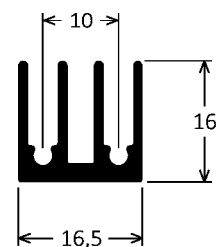
EE-119 0,320kg/m
