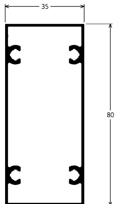
CX-102 1,024kg/m
