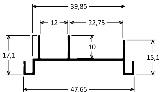
CX-350 0,231kg/m
