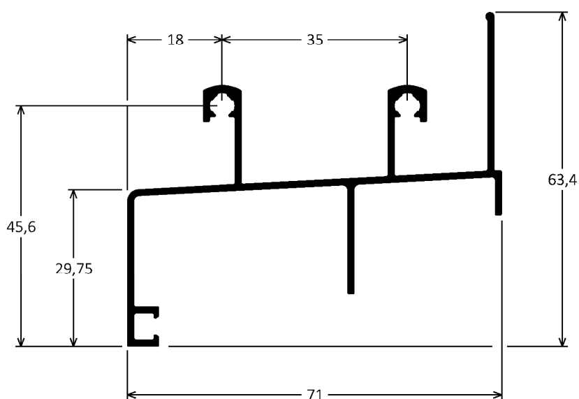
ISU-027 0,825kg/m
