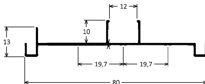
CX-979 0,311kg/m
