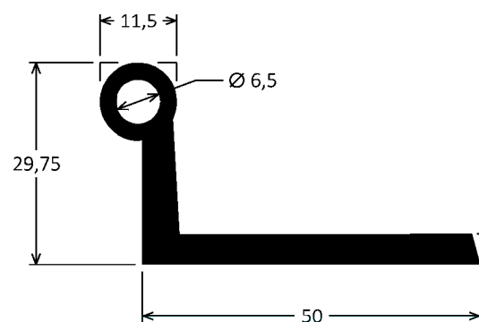
BK-333 0,997kg/m
