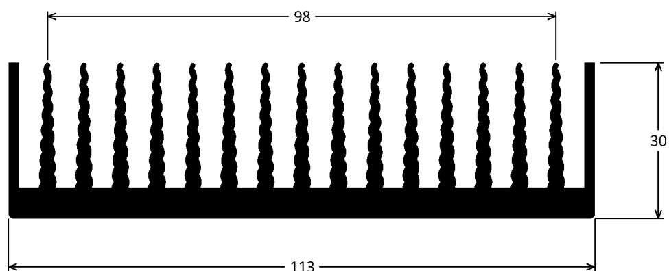
EE-059 4,196kg/m
