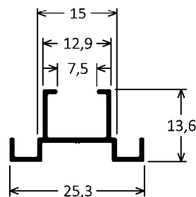
CX-470 0,149kg/m
