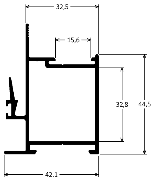
GI-048 0,890kg/m
