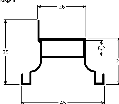
CX-015 0,410kg/m
