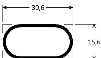
BK-189 0,263kg/m
