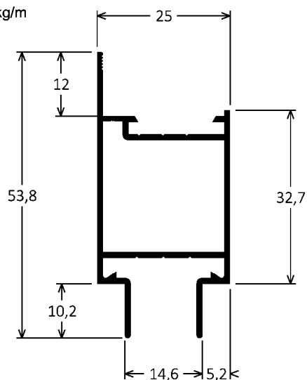
ISU-192 0,475kg/m
