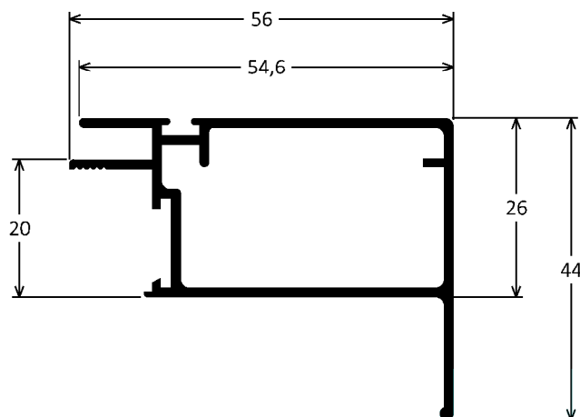
IMP-069 0,728kg/m
