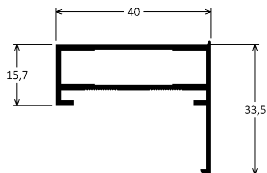
FC-261 0,516kg/m
