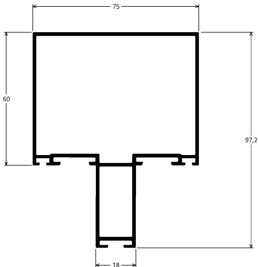
FC-202 1,691kg/m
