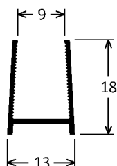
CX-055 0,115kg/m
