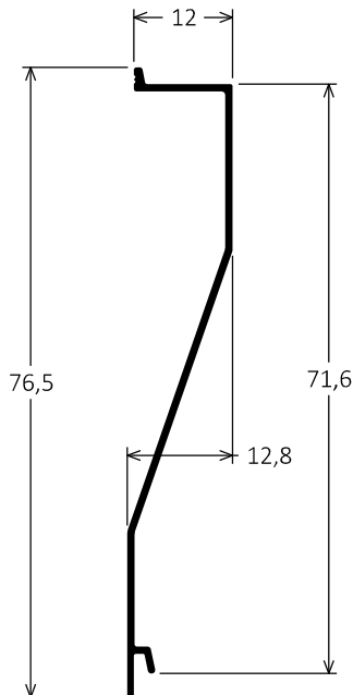
CX-517 0,230kg/m
