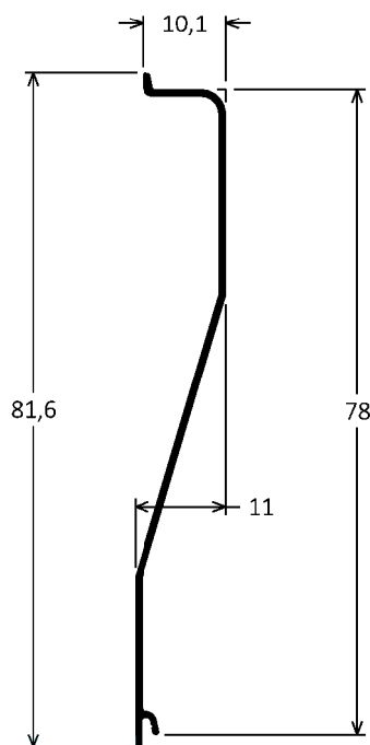
CX-140 0,228kg/m
