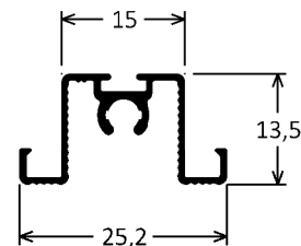
CX-170 0,174kg/m
