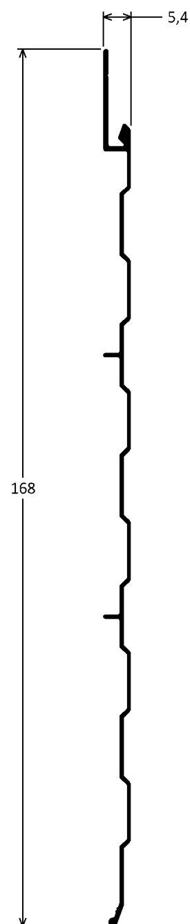
LB-010L 0,450kg/m
