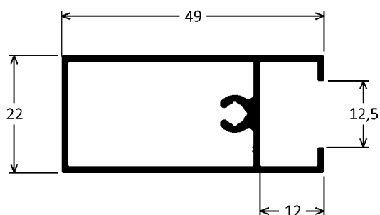
CX-999 0,535kg/m
