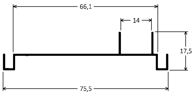
CX-519 0,297kg/m
