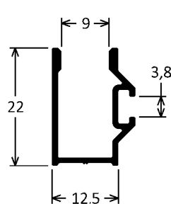
BX-224 0,200kg/m
