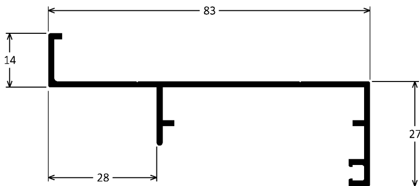
Z-118 0,618kg/m 30-039
