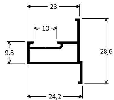
23-020 0,242kg/m ( BX-041)
