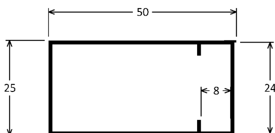
CX-011 0,411kg/m
