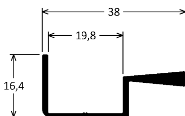
MV-046 0,277kg/m
