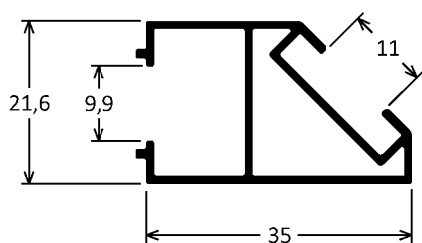
BK-187 0,368kg/m
