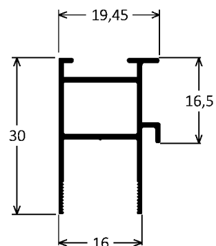
CX-118 0,270kg/m
