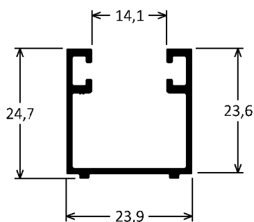
BX-143 0,310kg/m
