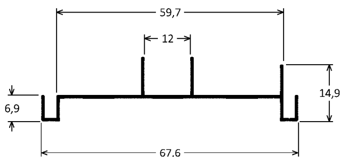
CX-347 0,271kg/m
