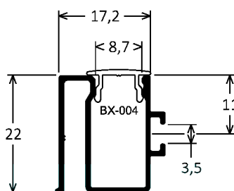
BX-333 0,241kg/m
