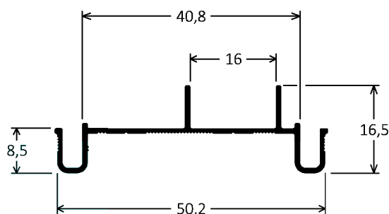
CX-523 0,250kg/m
