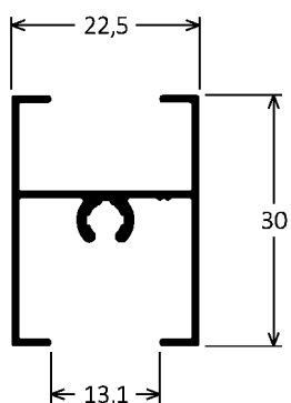
CX-042 0,282kg/m
