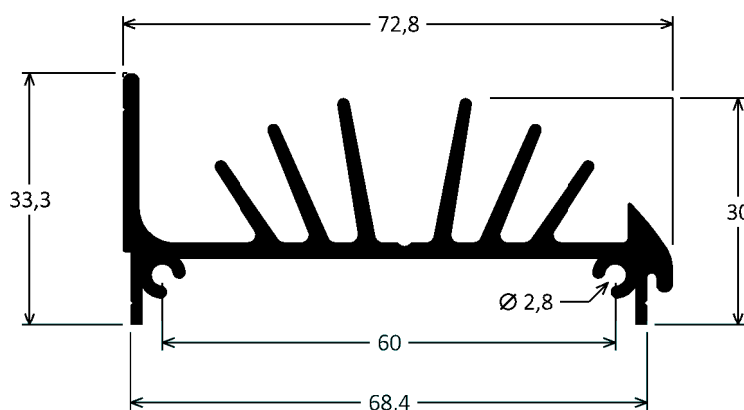
EE-062 1,296kg/m
