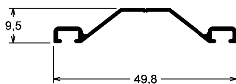
BK-626 0,211kg/m
