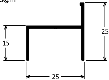
23-008 0,222kg/m
