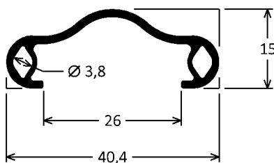
AP-012 0,305kg/m
