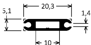
BK-186 0,156kg/m
