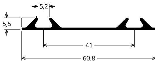
DV-107 0,282kg/m
