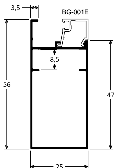
25-504E 0,372kg/m
