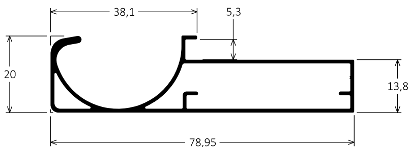
MMO-7575 0,613kg/m
