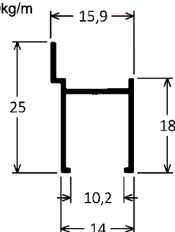
CX-521 0,159kg/m
