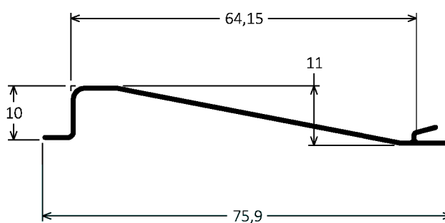
CX-779 0,220kg/m
