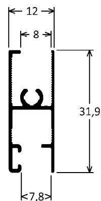
ISA-005 0,226kg/m
