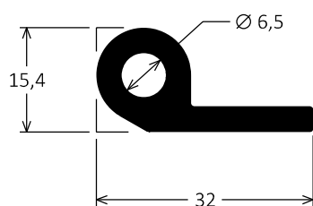
BK-182 0,570kg/m
