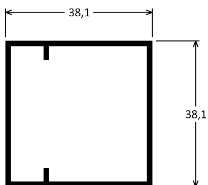
D-102 0,583kg/m
