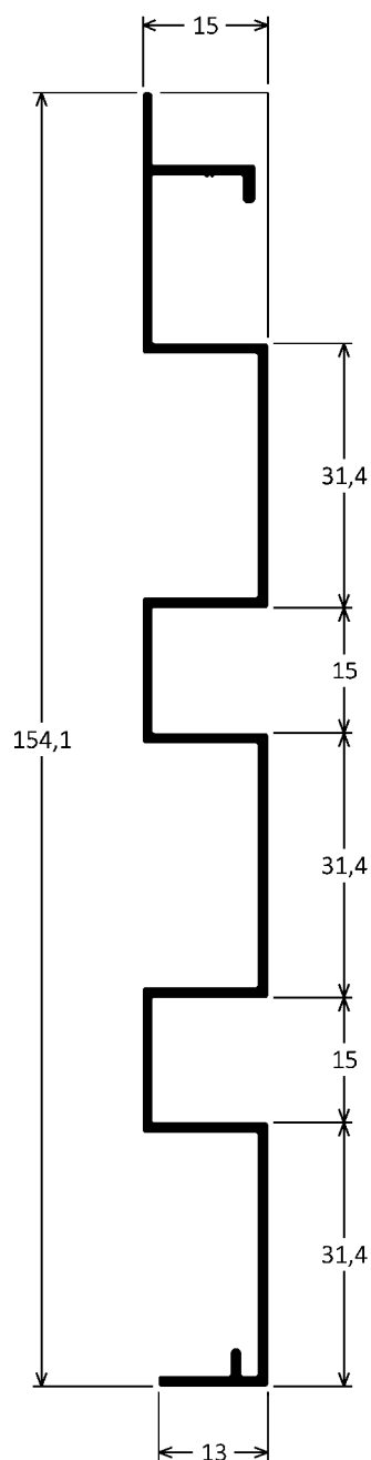
LB-175 0,827kg/m
