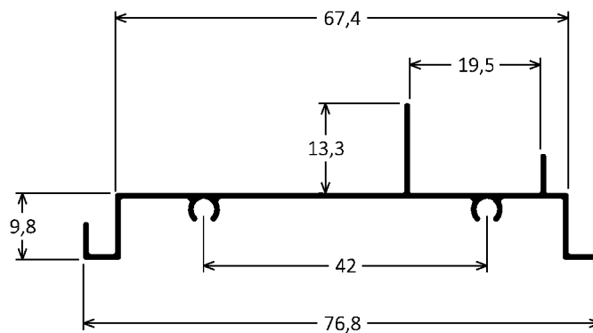
CX-424 0,301kg/m
