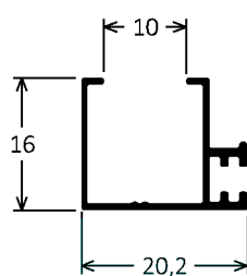
CX-030 0,149kg/m
