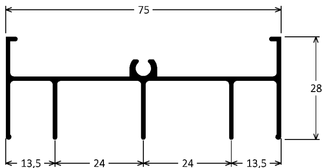
IMB-005 0,640kg/m
