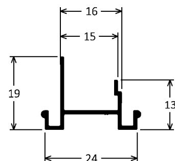
CX-027 0,179kg/m
