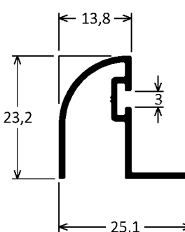
BX-006 0,236kg/m
