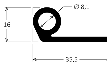
BK-090 0,447kg/m
