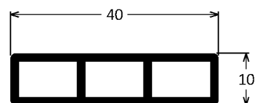
BK-015 0,462kg/m
