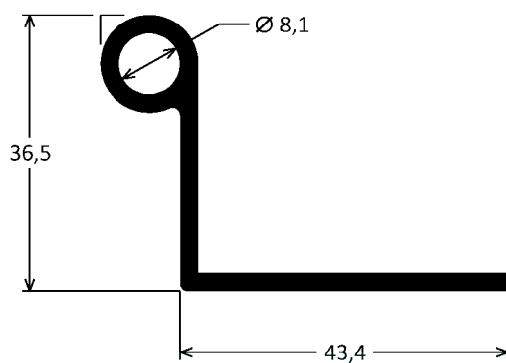
BK-089 0,660kg/m
