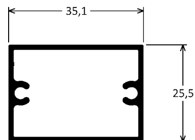
D-055 0,490kg/m
