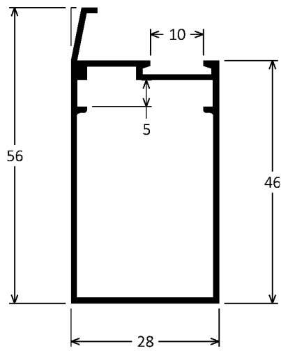
P-530 0,514kg/m
