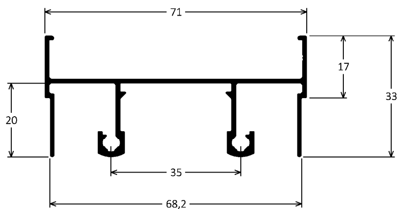
ISU-001 0,718kg/m
