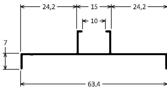
CX-571 0,235kg/m
