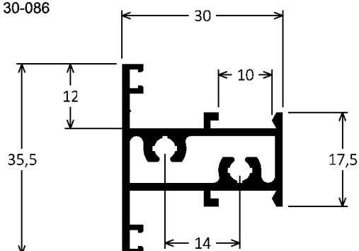
P-075 0,599kg/m 30-086
