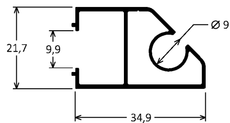
BK-188 0,355kg/m
