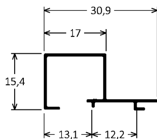
CX-428 0,156kg/m
