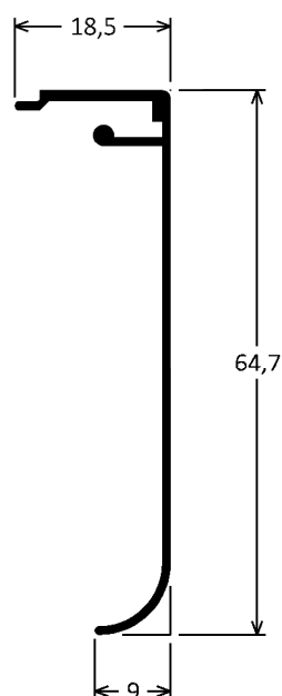
BX-130 0,286kg/m
