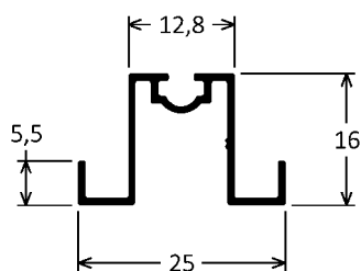
CX-557 0,178kg/m
