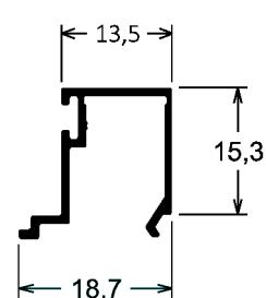
GI-057 0,159kg/m
