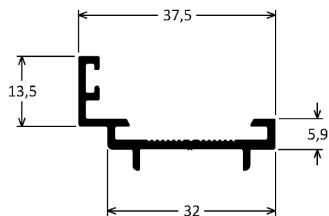
GI-016 0,331kg/m
