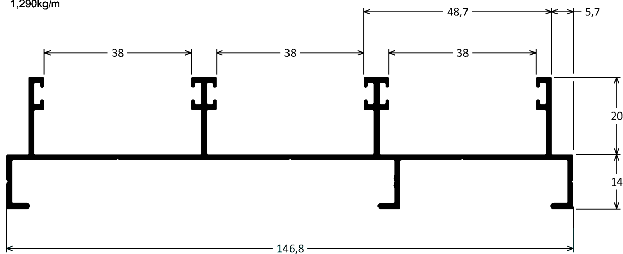
GI-064 1,290kg/m
