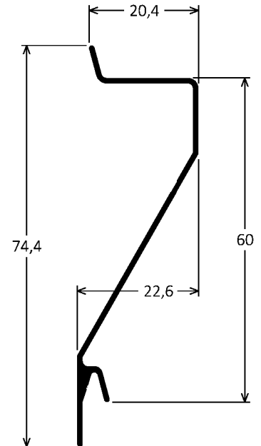
Z-203 0,301kg/m
