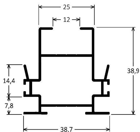
ISU-057 0,591kg/m
