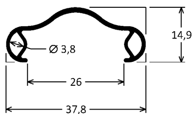
AP-051 0,232kg/m
