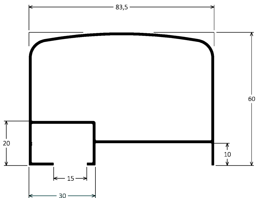
ICG-072 1,017kg/m
