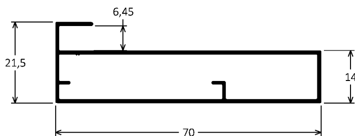
MMO-011 0,539kg/m
