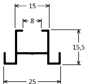
CX-554 0,166kg/m
